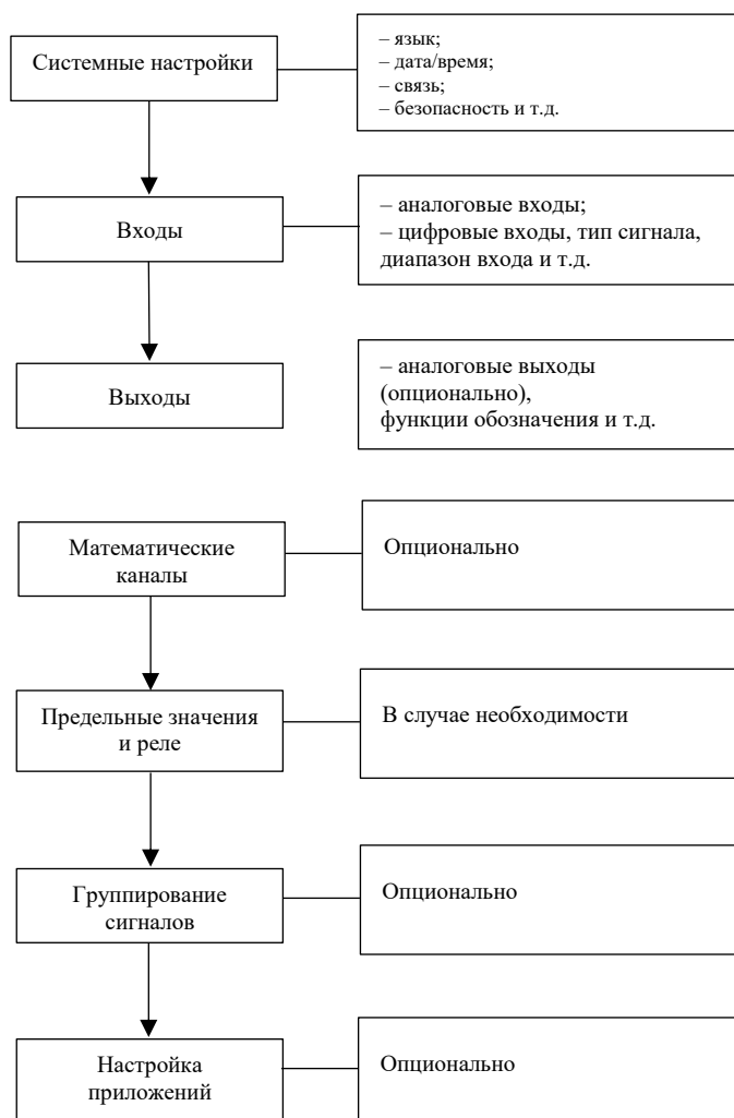
Рисунок 2.1 – Последовательность настройки прибора
