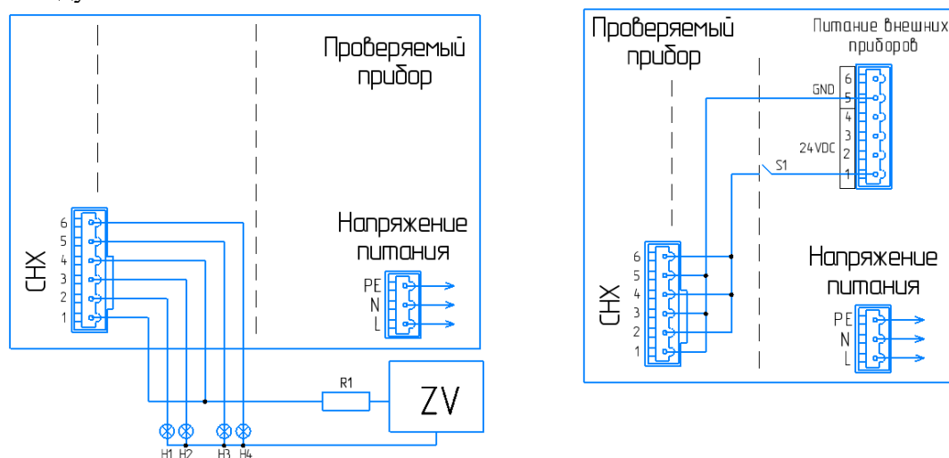
Рисунок Г.5 – Определение основной погрешности преобразования прибора «Мультиграф» по токовому выходу
