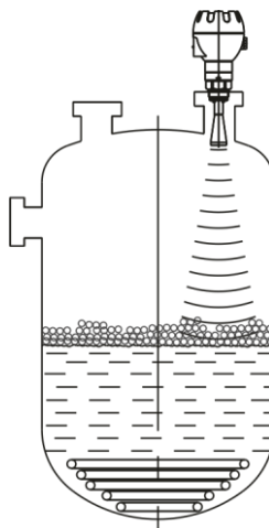
Рисунок 5 – Пенообразование
