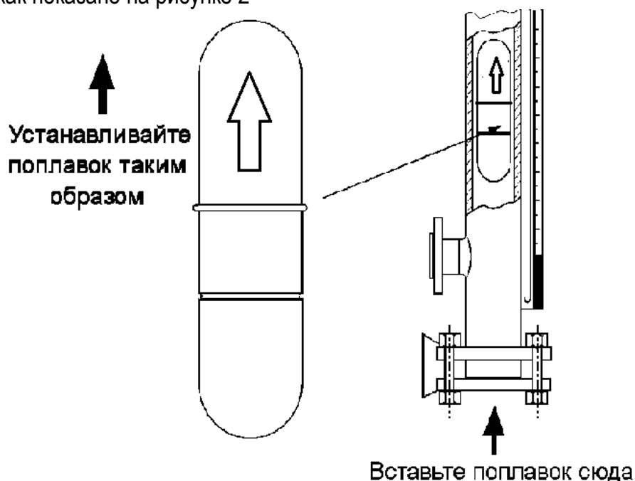
Рисунок 2 – Установка поплавка
