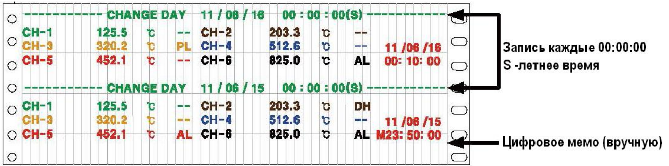
Рисунок 26 – Пример записи в цифровом режиме
