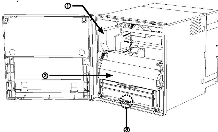
Рисунок 5 – Вид прибора с открытой крышкой
