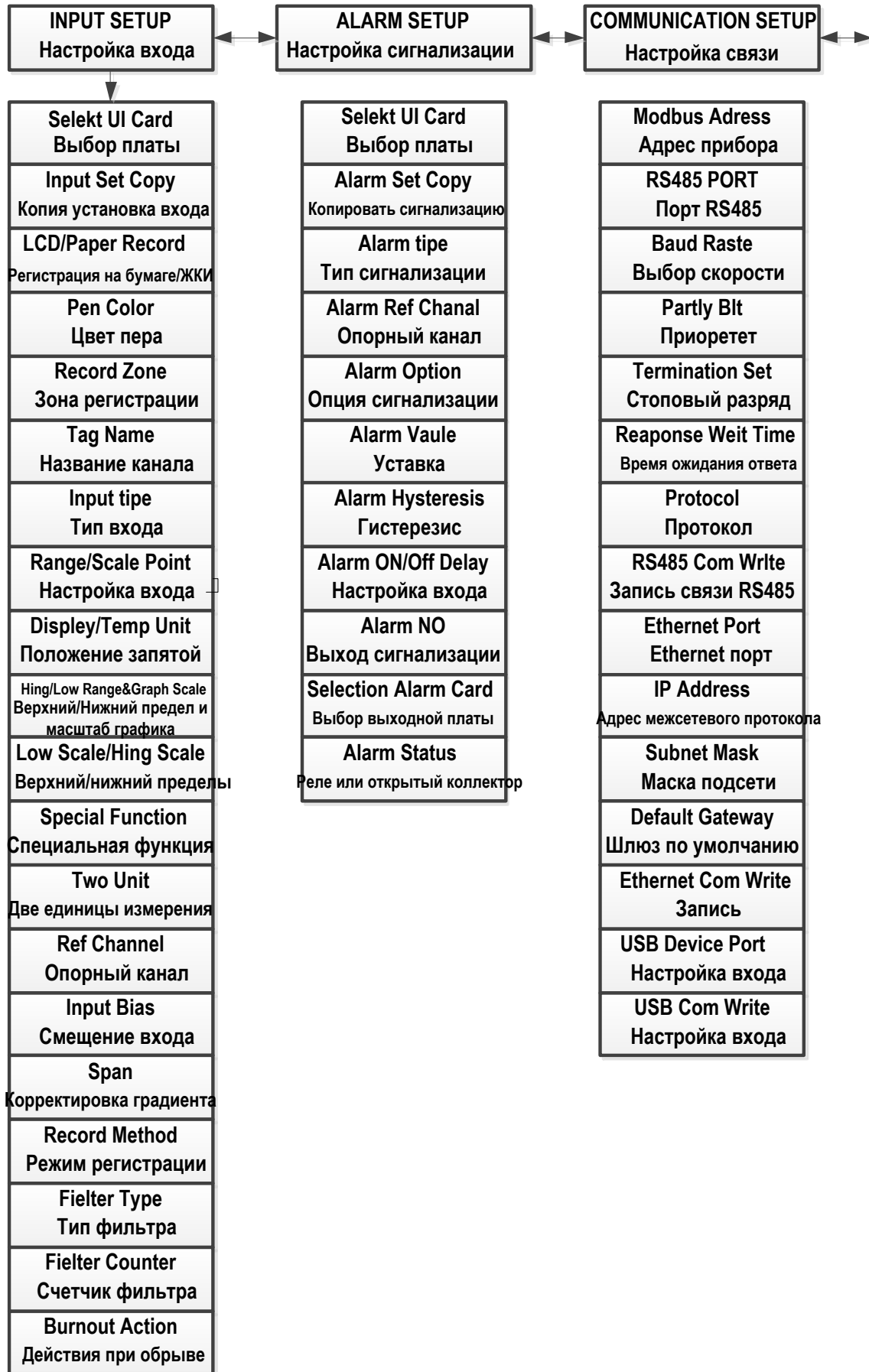
Рисунок 20.1 – Состав параметров для настройки прибора (продолжение рисунок 20.2)
