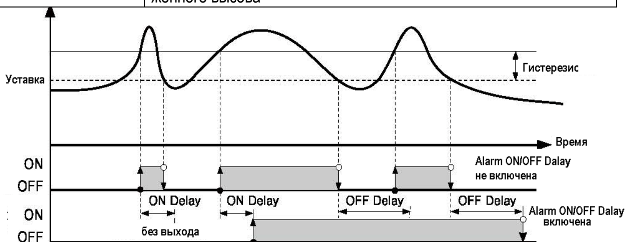
Рисунок 24– Пример работы сигнализации при включении/выключении Alarm On/OFF Delay
