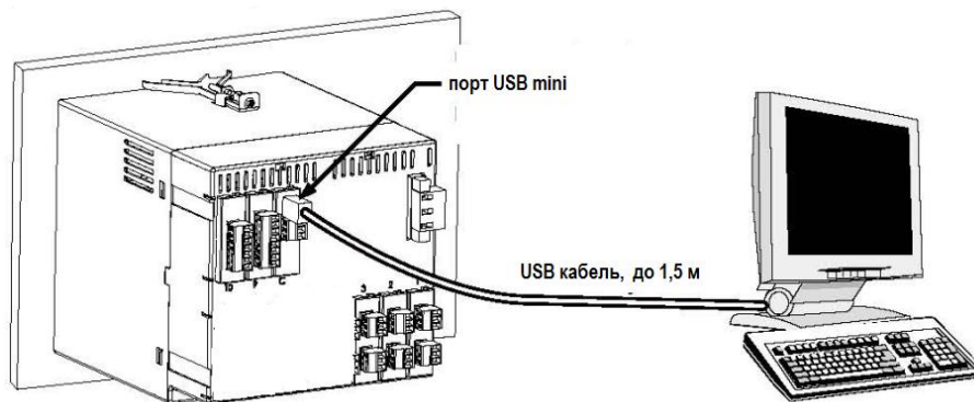
Рисунок 12 – Подключение прибора к персональному компьютеру
