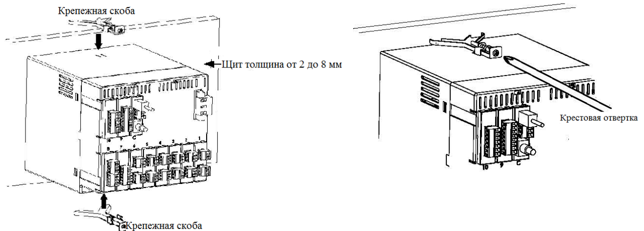
Рисунок 7.1 – Установка прибора в щит Рисунок 7.2 – Закрепление прибора в щите
