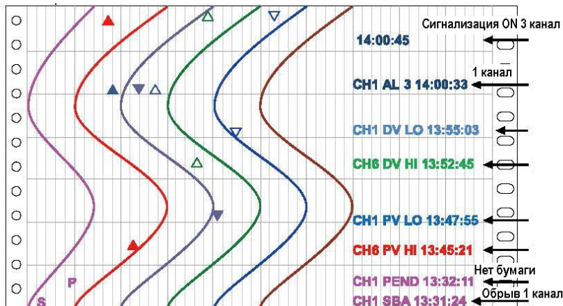
Рисунок 21 – Пример 1 регистрации срабатывания сигнализации в графическом режиме
