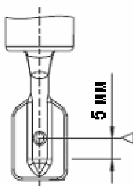
Монтаж сверху
